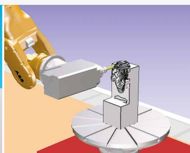
Fräsen mit realistischer Abtragssimulation
